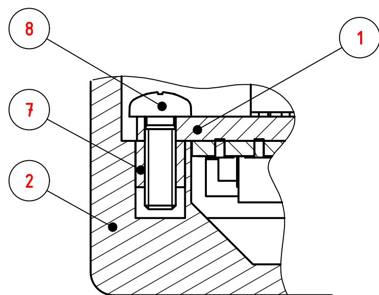
DETALLE B (4 : 1)
